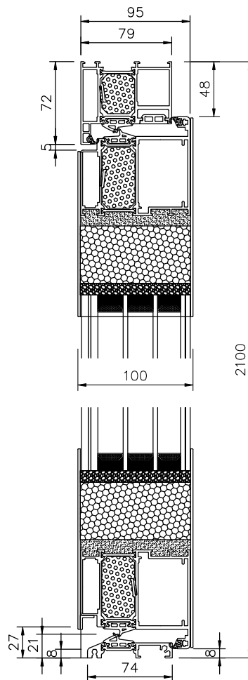
Arcade 79 mm Türrahmen bündig mit Flügelprofil
